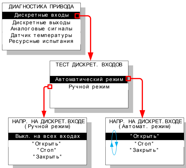
Рисунок 9 – Структура подменю "Диагностика привода"– "Тест.дискрет.входов"
